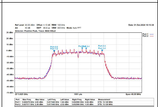
802.11a / Ant.1+Ant.2 / 6M / 5825MHz / Ch165
