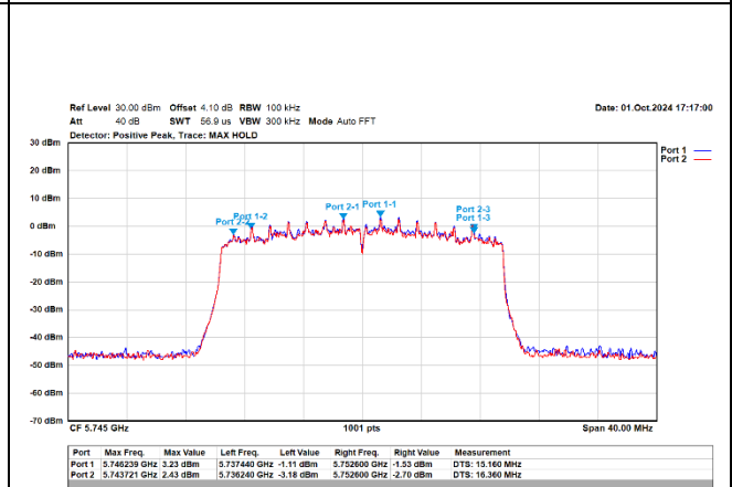
802.11be / 20MHz / Ant.1+Ant.2 / MCS0 / 5745MHz / Ch149
