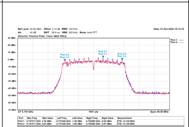
802.11a / Ant.1+Ant.2 / 6M / 5745MHz / Ch149
