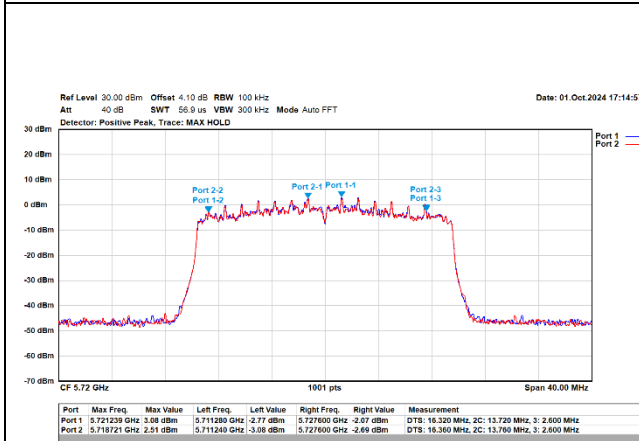
802.11be / 20MHz / Ant.1+Ant.2 / MCS0 / 5720MHz / Ch144
