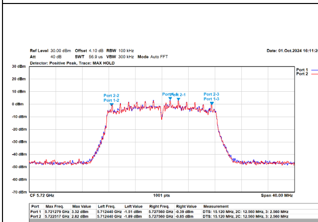
802.11a / Ant.1+Ant.2 / 6M / 5720MHz / Ch144
