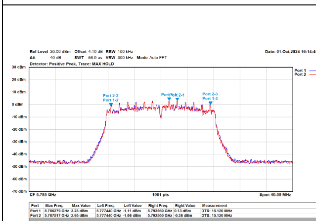
802.11a / Ant.1+Ant.2 / 6M / 5785MHz / Ch157
