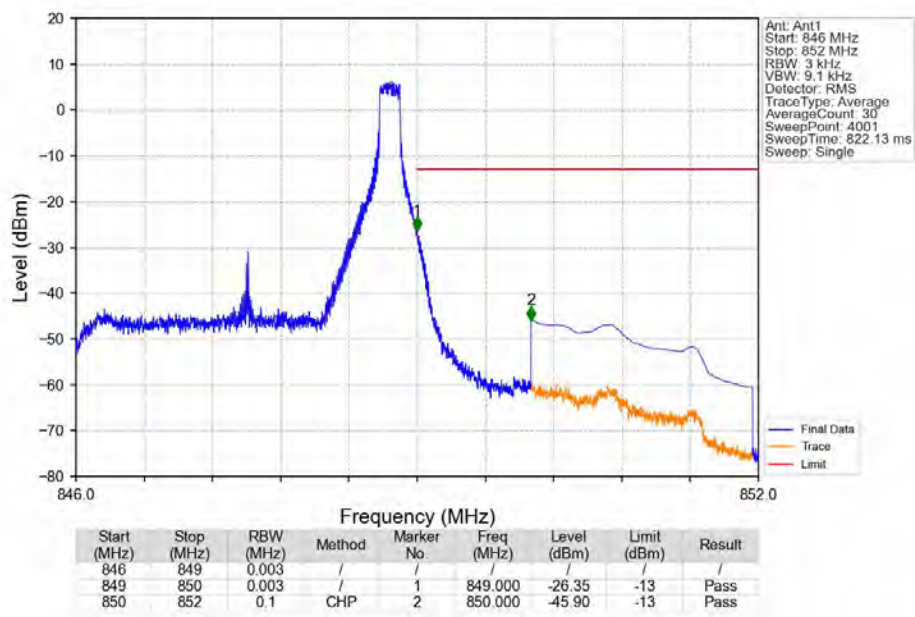
Band5_3MHz_QPSK_HCH_847.5MHz_RB_1_14_NTNV
