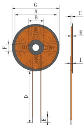
一、尺寸 DIMENSION:(mm)
