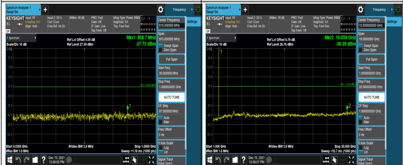
Band4-1.4MHz-QPSK-20393-1RB#0-Range1:30~1000MHz
