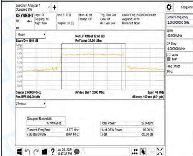
41(2555-2655)-20MHz-16QAM-40690-100RB#0-PASS
