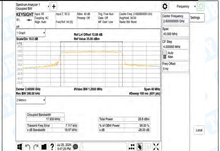
41(2555-2655)-20MHz-16QAM-40340-100RB#0-PASS
