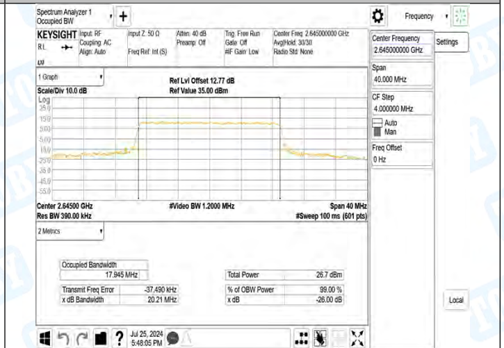
41(2555-2655)-20MHz-16QAM-41140-100RB#0-PASS
