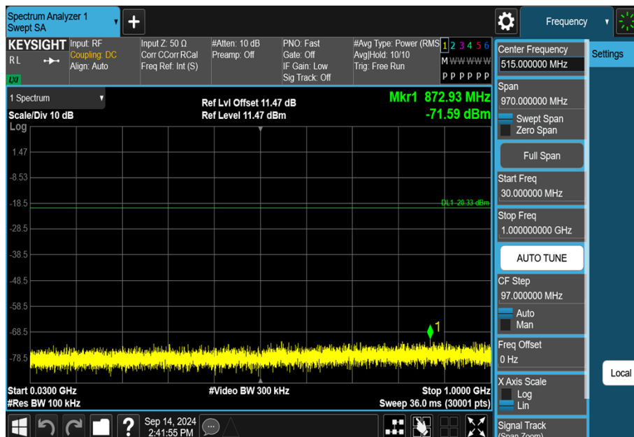
11G-Ant1-2462-30~1000-PASS
