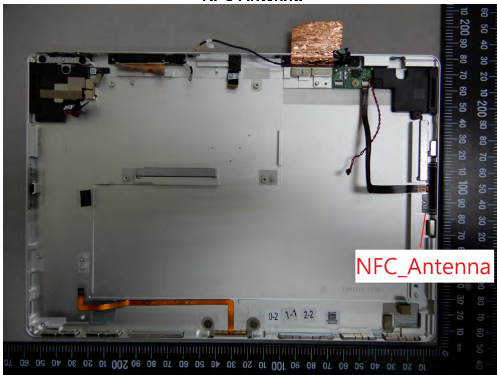
NFC Antenna
