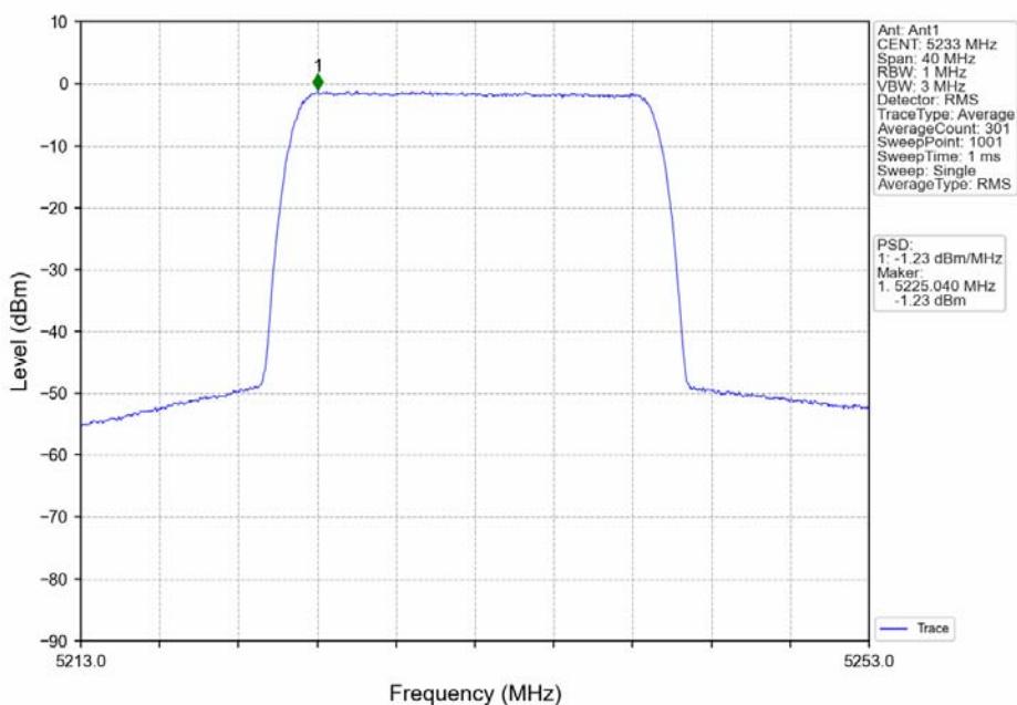
16QAM 20MHz_HCH_5233MHz_Ant1_NTNV
