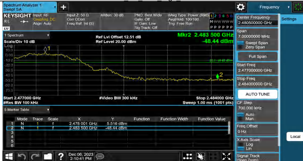
BLE 2M Ant1 High 2478
