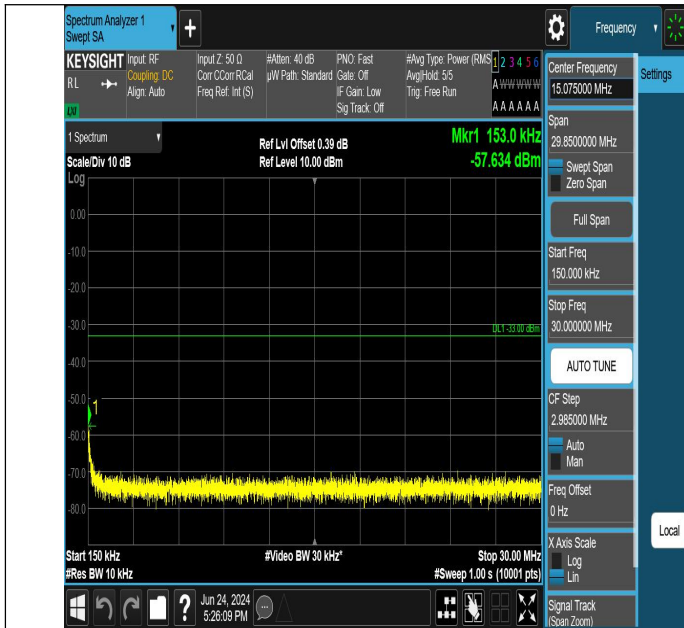
GSM1900-661-0-0.15~30MHz-PASS
