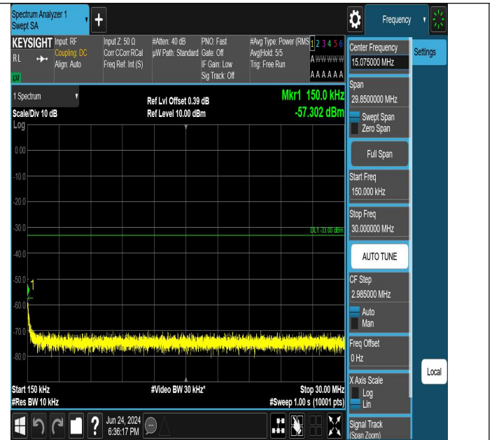
GPRS1900-661-0-0.15~30MHz-PASS
