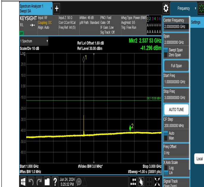
GSM1900-512-0-1000~3000MHz-PASS
