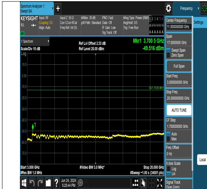
GSM1900-512-0-3000~20000MHz-PASS
