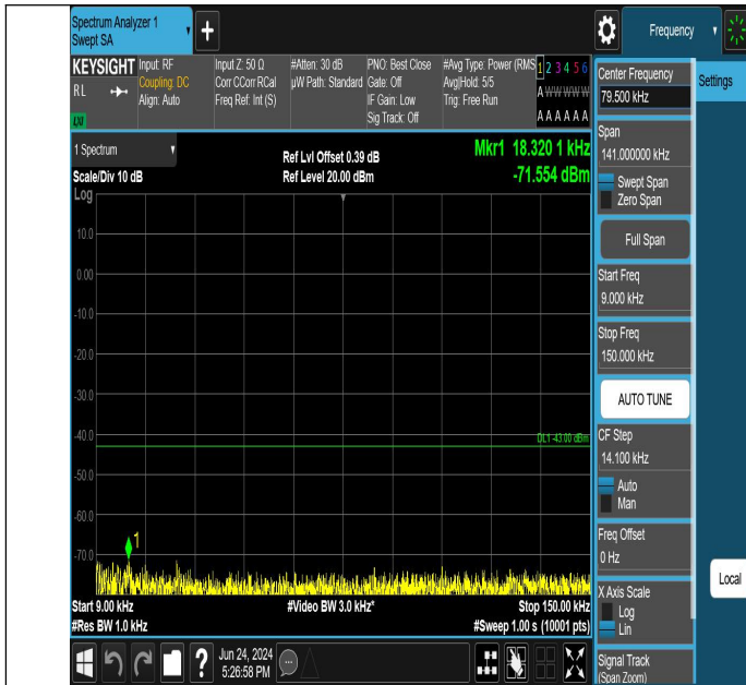
GSM1900-810-0-0.009~0.15MHz-PASS
