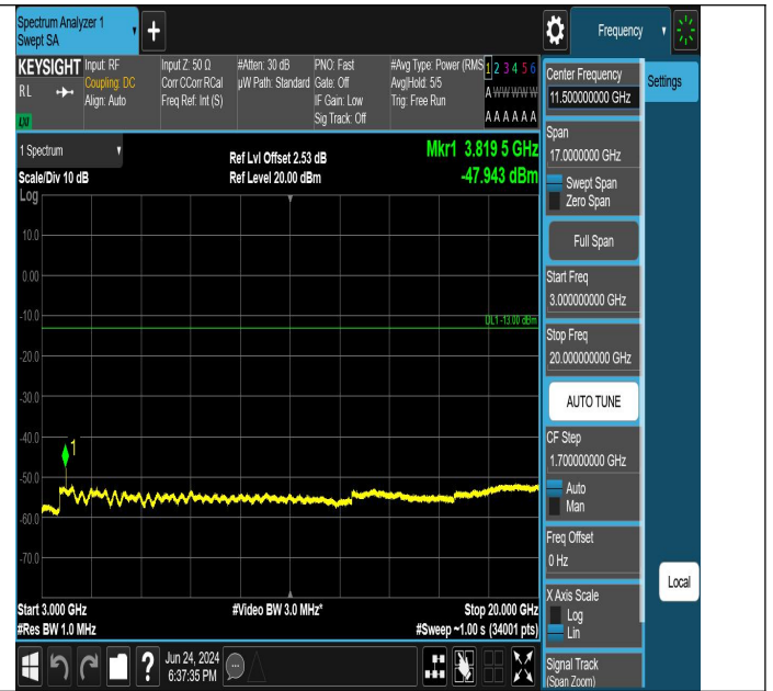
GPRS1900-810-0-3000~20000MHz-PASS
