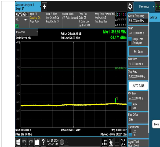
GSM1900-512-0-30~1000MHz-PASS
