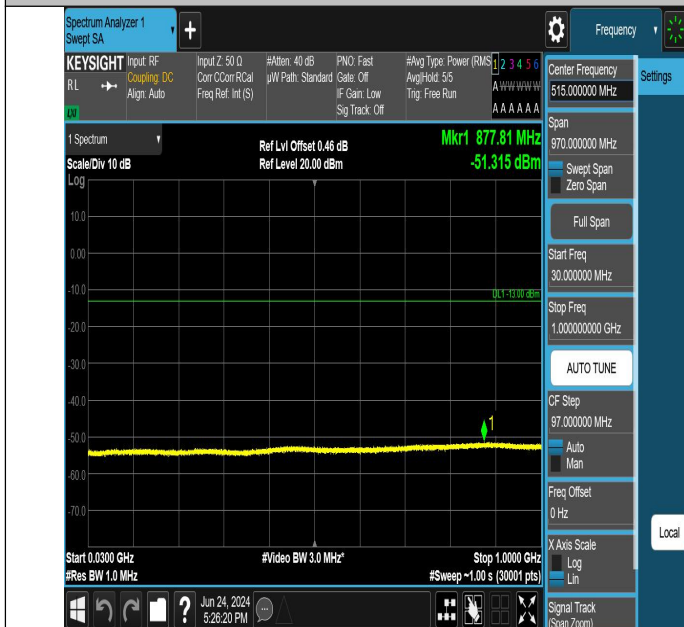
GSM1900-661-0-30~1000MHz-PASS
