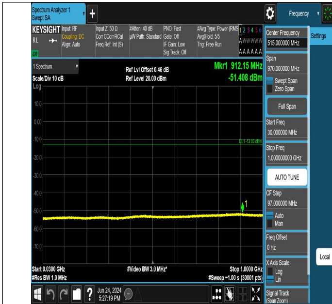
GSM1900-810-0-30~1000MHz-PASS
