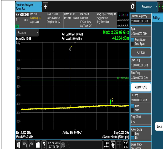
GSM1900-810-0-1000~3000MHz-PASS
