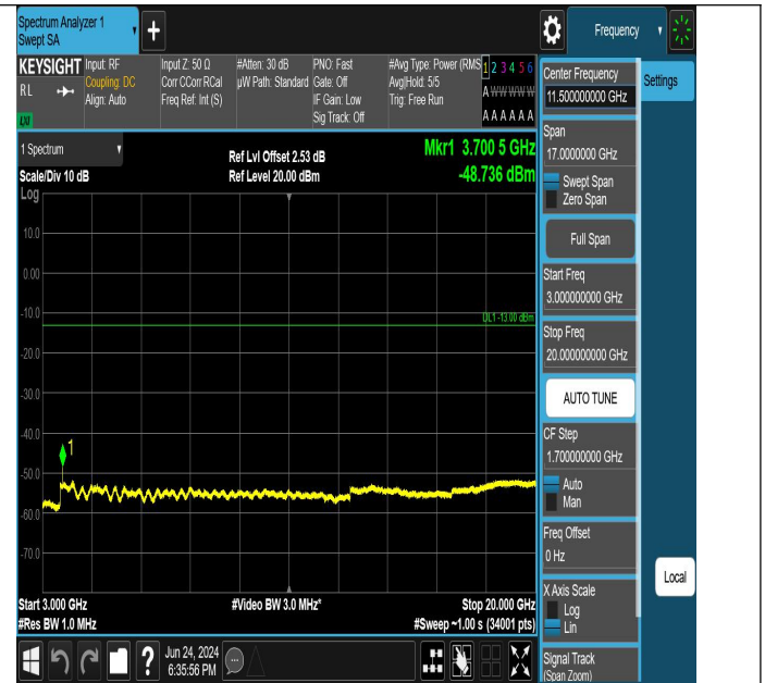
GPRS1900-512-0-3000~20000MHz-PASS
