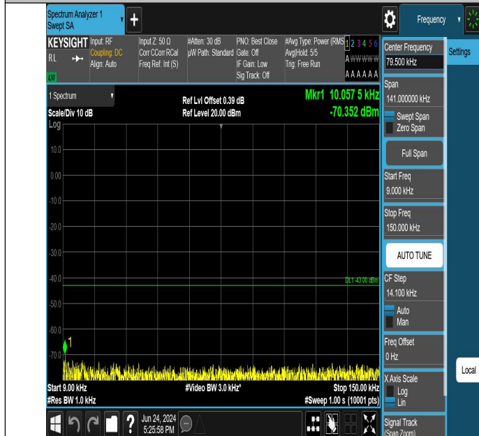
GSM1900-661-0-0.009~0.15MHz-PASS
