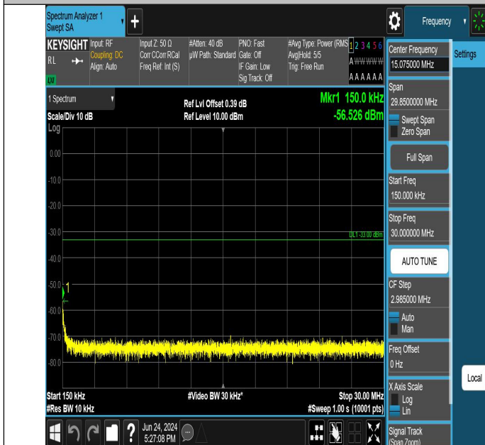
GSM1900-810-0-0.15~30MHz-PASS
