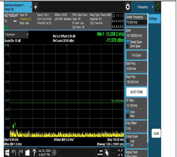
GPRS1900-661-0-0.009~0.15MHz-PASS
