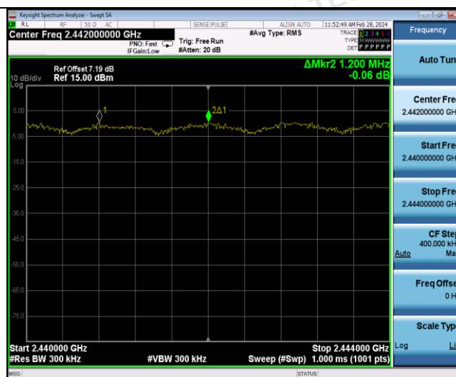
\pi/4\text{DQPSK}
