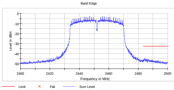
Band Edge Ch09 802.11n HT40 MCS8 MIMO
