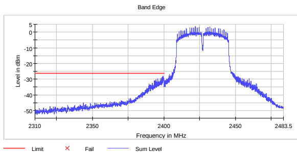
Band Edge Ch04 802.11n HT40 MCS8 MIMO
