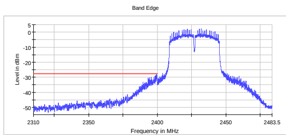
Band Edge Ch03 802.11n HT40 MCS0 SISO
