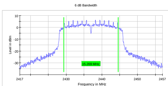
DTS BW, 2437 MHz, 802.11n SISO MCS0
