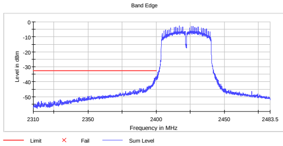
Band Edge Ch03 802.11n HT40 MCS8 MIMO
