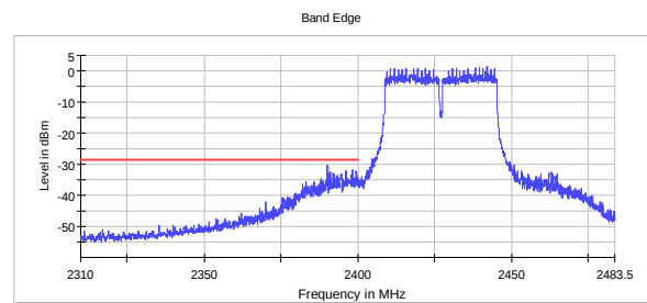
Band Edge Ch03 802.11n HT40 MCS7 SISO
