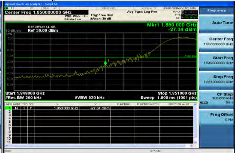
Band Edge_Band2 15MHz_QPSK 1 0_LowCH18675-1857.5
