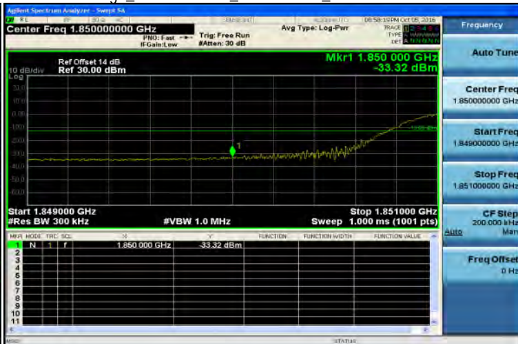
Band Edge_Band2 20MHz_QPSK 100 0_LowCH18700-1860
