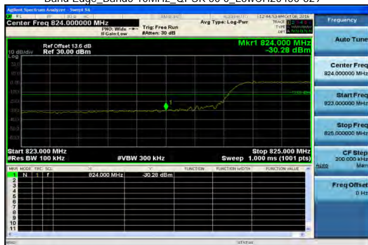
Band Edge_Band5 10MHz_QPSK 50 0_LowCH20450-829
