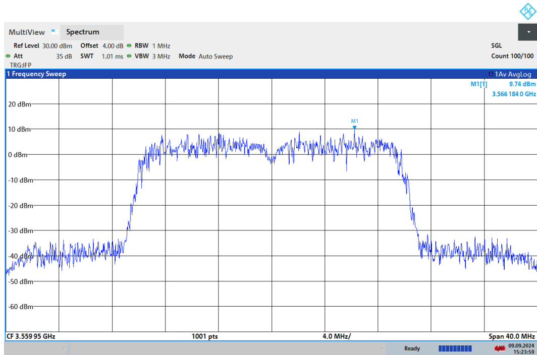
CA_48B 256QAM\10MHz+10MHz Low
