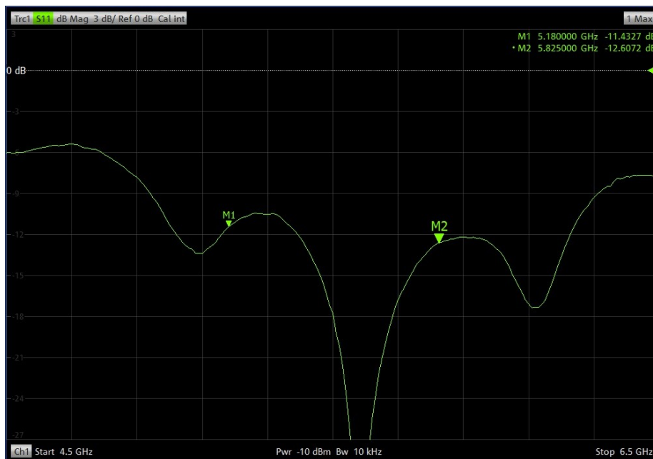
Antenna 3 (5 GHz / ch0)
