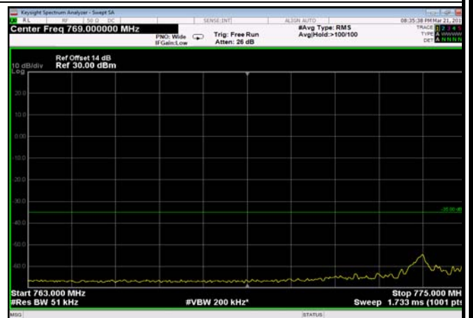
FDD13_5MHz_784.5_QPSK_OneRB_low _ExtraBands_Range_763~775
