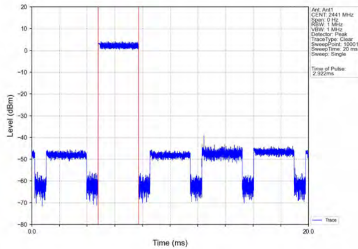
8DPSK_3DH5_HOPP_Ant1_NTNV
