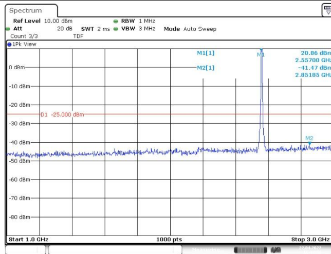
Band41-5MHz-QPSK-40265-25RB#0-Range2:1000~3000MHz
