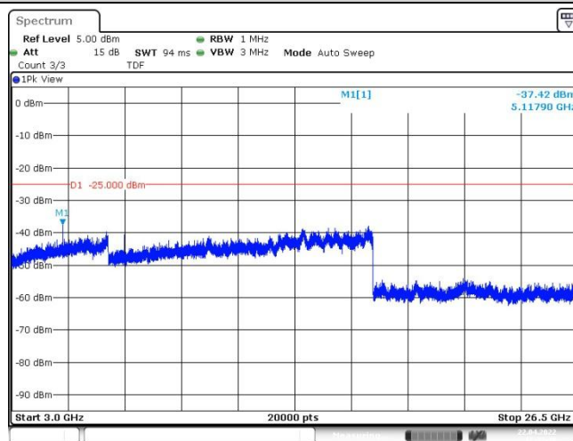
Band41-5MHz-QPSK-40265-25RB#0-Range3:3000~26500MHz
