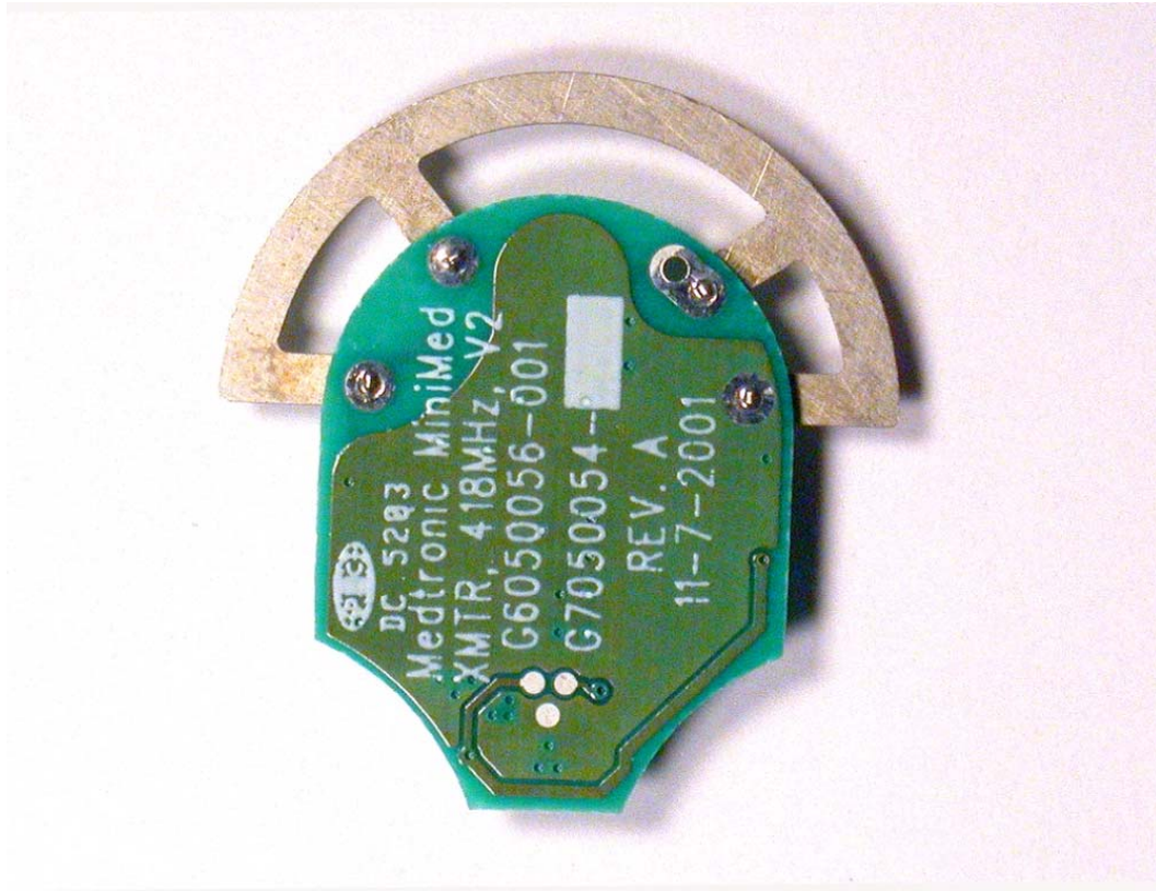
PCB TOP 2
