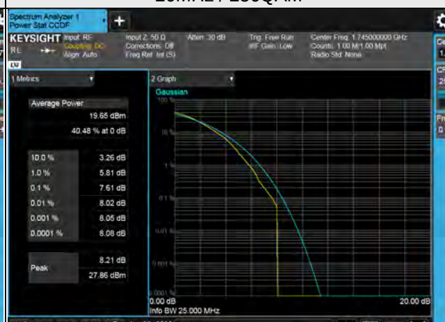
20MHz / 256QAM
