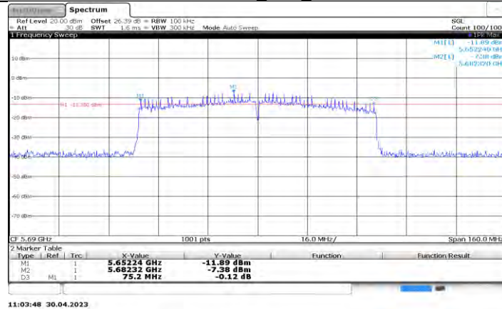
11AC80SISO_Ant1_5690
