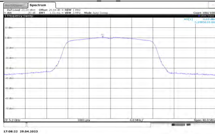
11A_Ant1_5200
