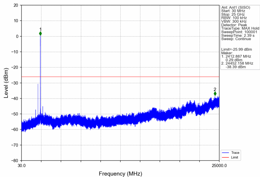
802.11ax(HEW20) LCH 2412MHz RU242 Left Ant1 (SISO) NTN
