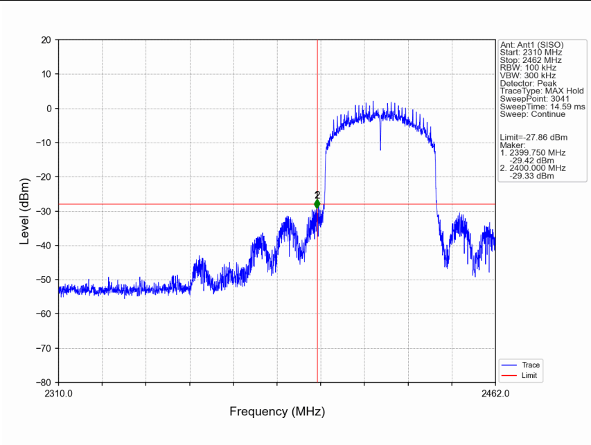
802.11ax(HEW40) LCH 2422MHz RU484 Left Ant1 (SISO) NTN
