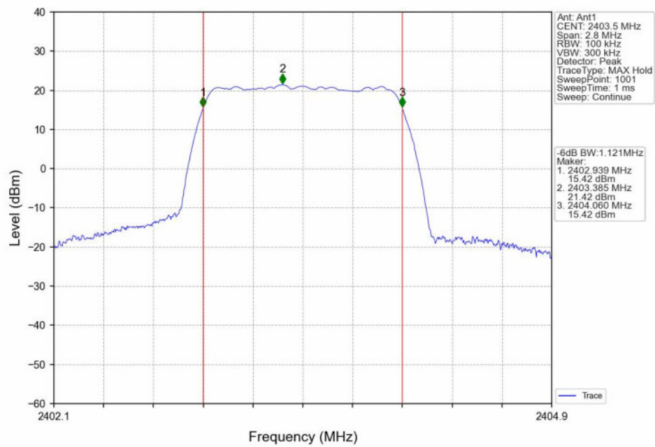
16QAM_LCH_2403.5MHz_MIMO_NTNV
