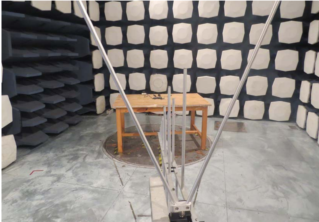
30MHz ~ 1GHz
