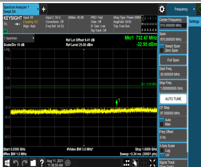
Band25-20MHz-QPSK-26365-1-0-Low-30-1000--32.95-PASS
