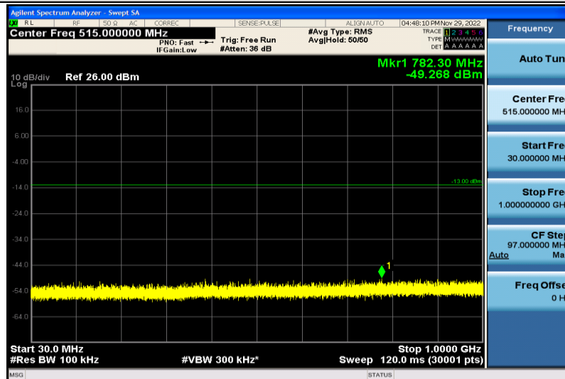
Band66-20MHz-QPSK-132572-1RB#0-30~1000MHz
