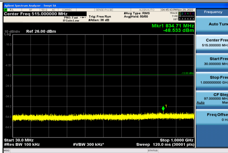
Band66-20MHz-QPSK-132072-1RB#0-30~1000MHz
