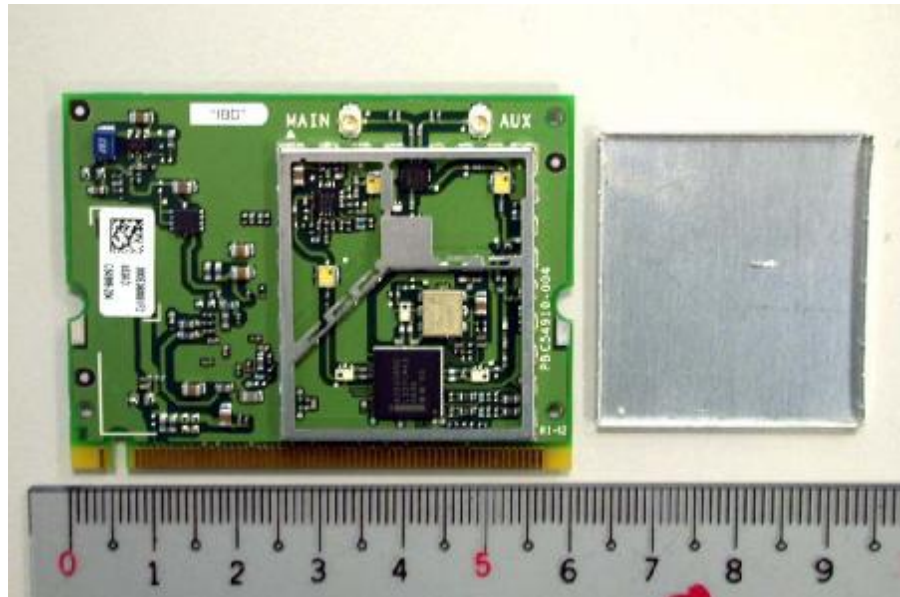
RF Module 1
