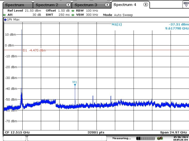
Zigbee Ant1 2405 30~25000
