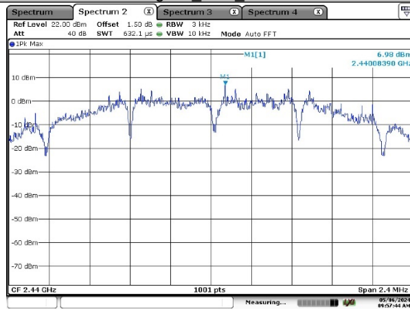
Zigbee Ant1 2440
