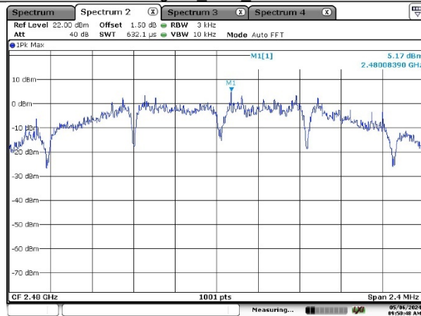
Zigbee Ant1 2480
