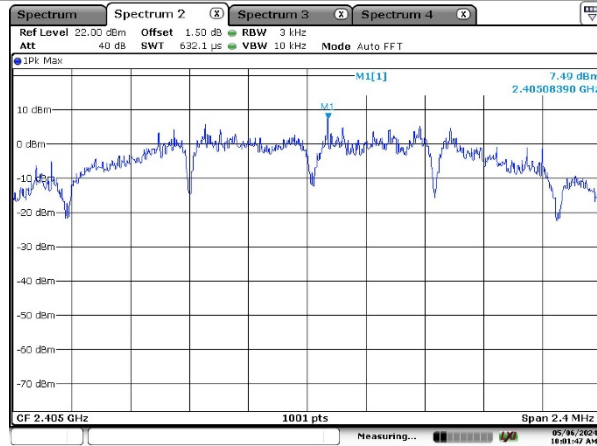
Zigbee Ant1 2405
