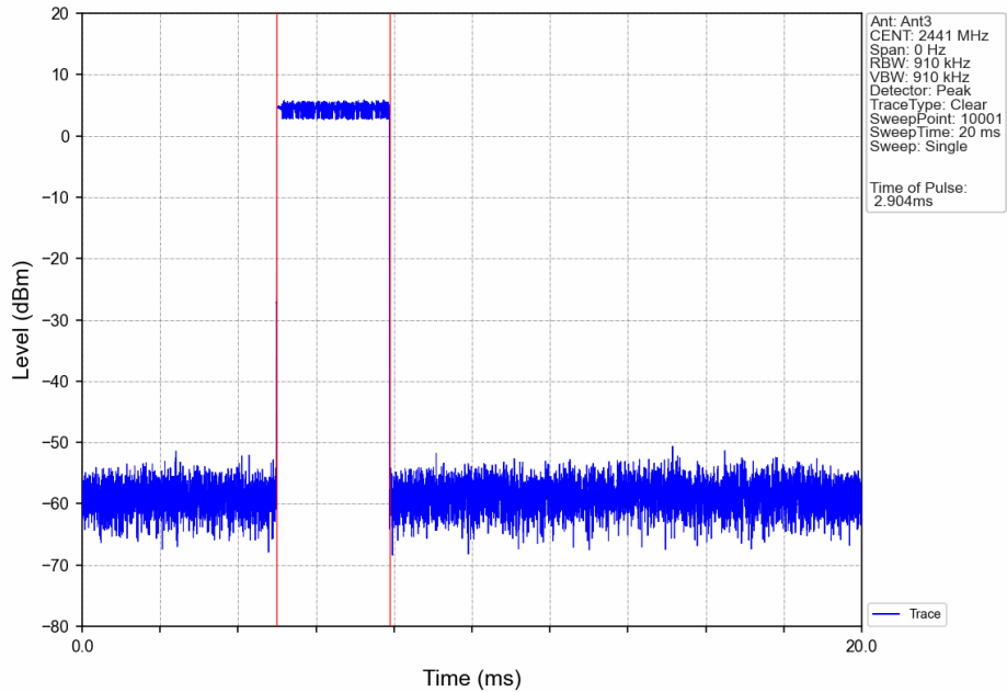
Pi/4DQPSK_2DH5_HOPP_Ant3_NTNV
