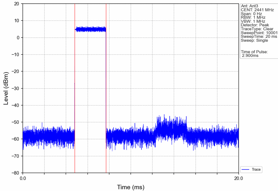
8DPSK_3DH5_HOPP_Ant3_NTNV
