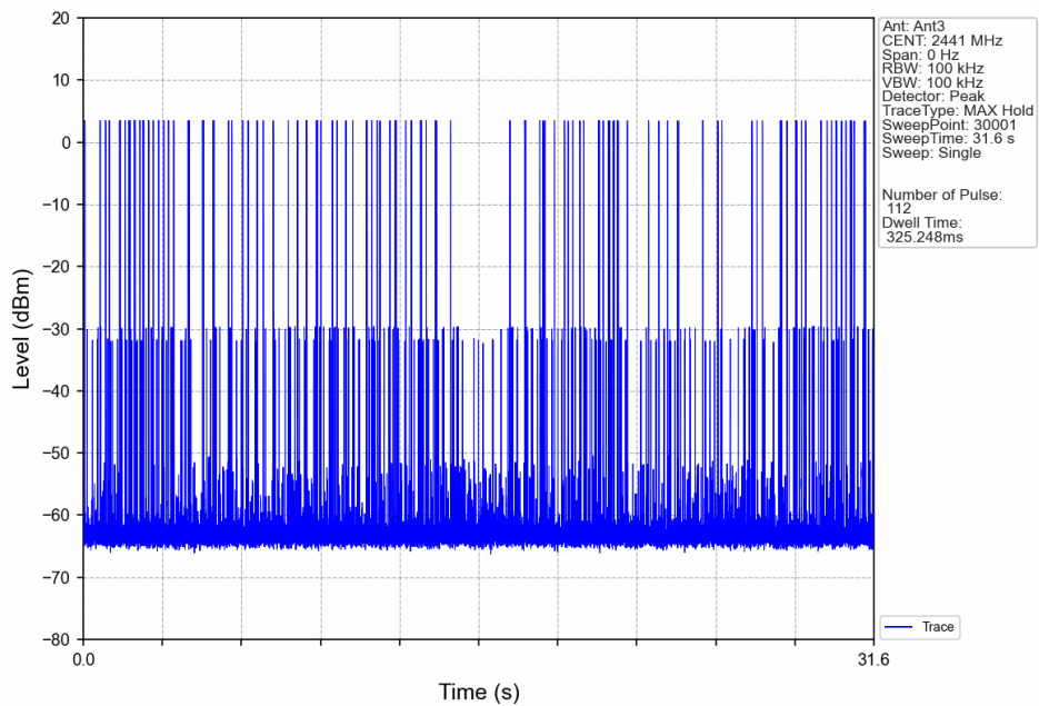
Pi/4DQPSK_2DH5_HOPP_Ant3_NTNV
