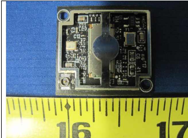
EUT - Top
