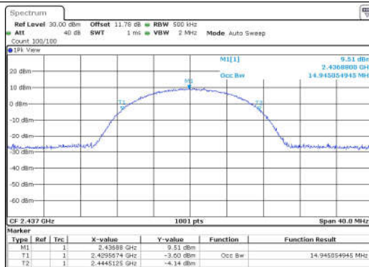
11B-Ant1-2437
