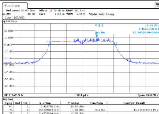
11G-Ant1-2462
