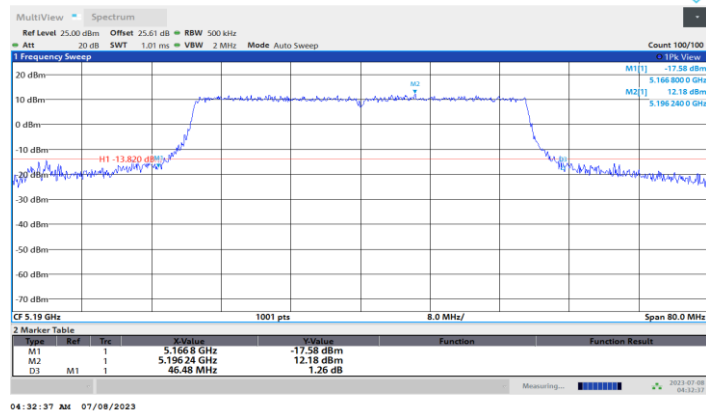
11BE40MIMO_Ant1_5190
