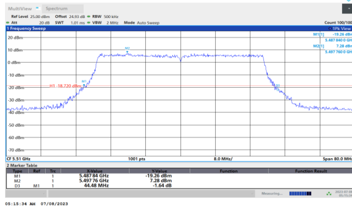
11BE40MIMO_Ant3_5510
