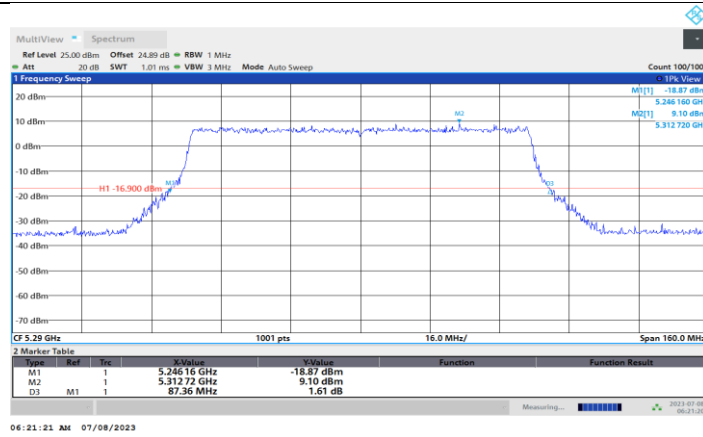
11BE80MIMO_Ant3_5290
