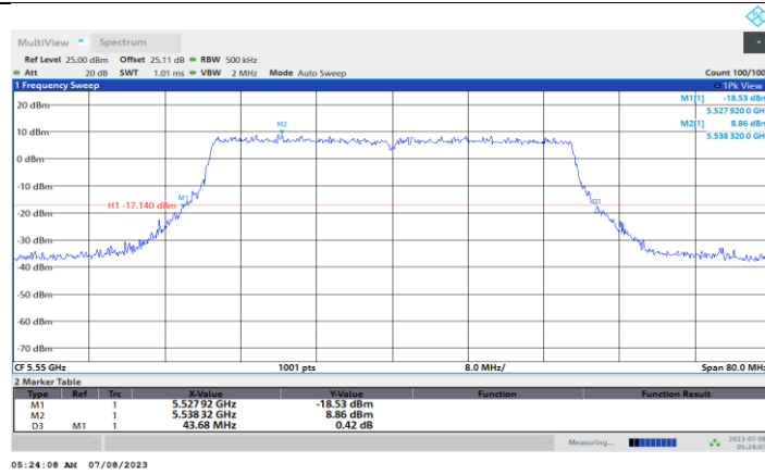
11BE40MIMO_Ant3_5550
