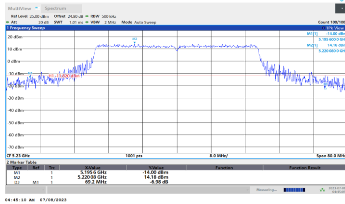
11BE40MIMO_Ant3_5230
