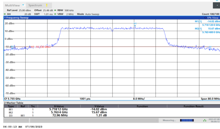
11BE40MIMO_Ant4_5755
