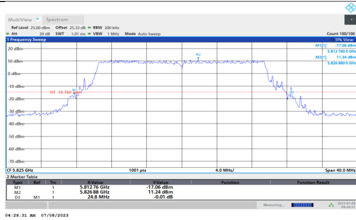
11BE20MIMO_Ant3_5825
