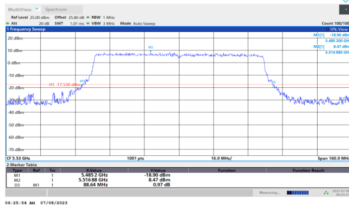
11BE80MIMO_Ant1_5530
