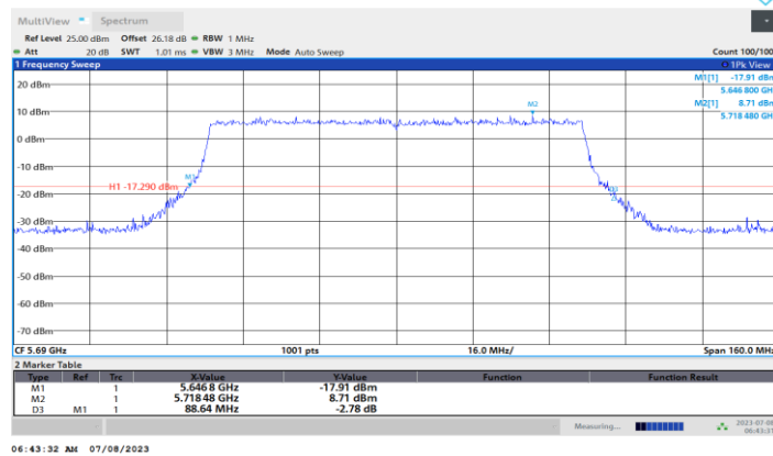
11BE80MIMO_Ant2_5690
