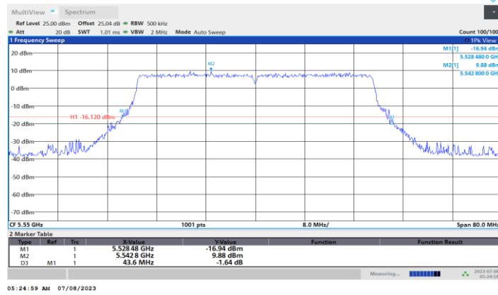
11BE40MIMO_Ant4_5550
