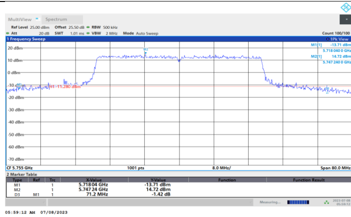
11BE40MIMO_Ant3_5755
