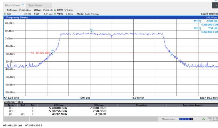
11BE40MIMO_Ant1_5310
