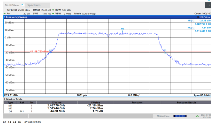
11BE40MIMO_Ant2_5510
