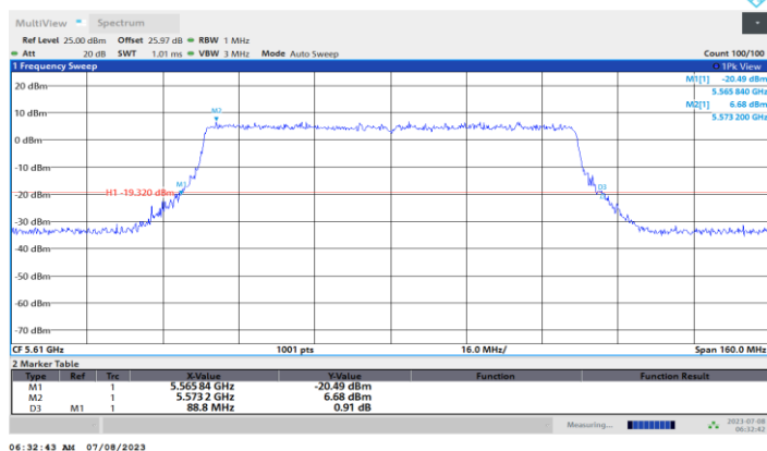
11BE80MIMO_Ant2_5610
