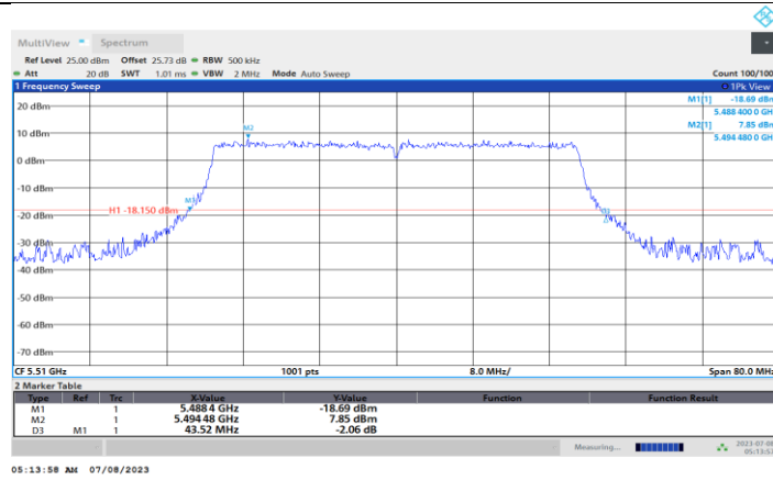
11BE40MIMO_Ant1_5510
