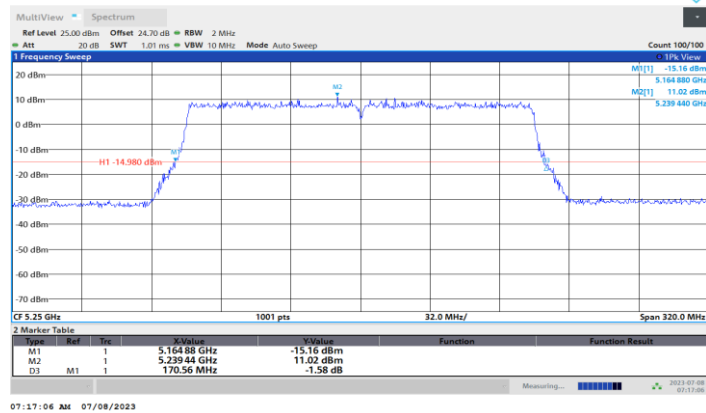
11BE160MIMO_Ant3_5250
