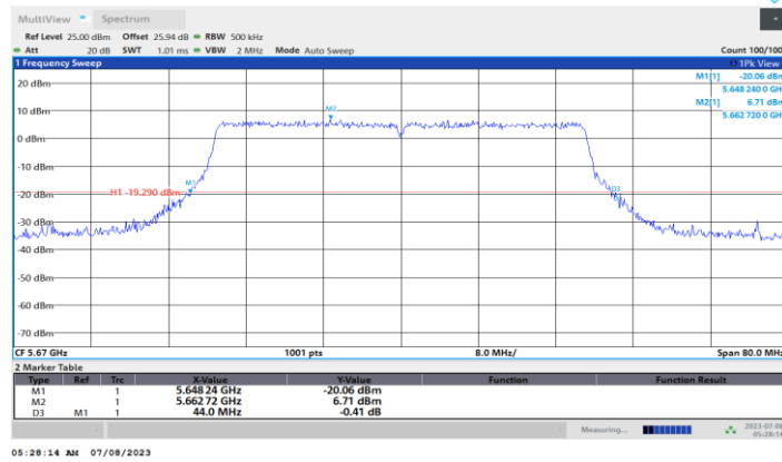
11BE40MIMO_Ant1_5670
