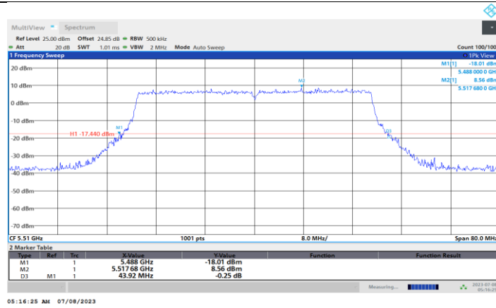
11BE40MIMO_Ant4_5510
