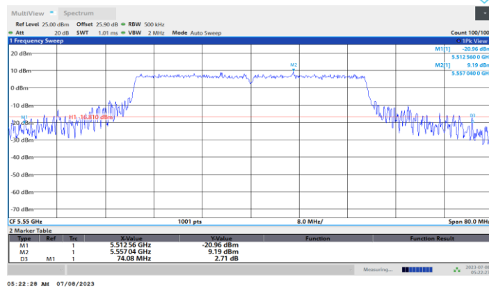
11BE40MIMO_Ant1_5550
