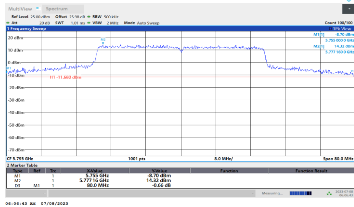
11BE40MIMO_Ant1_5795
