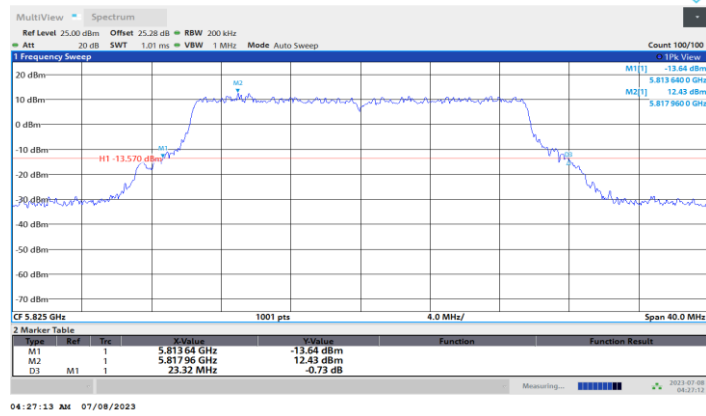
11BE20MIMO_Ant4_5825
