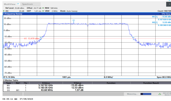
11BE40MIMO_Ant4_5190
