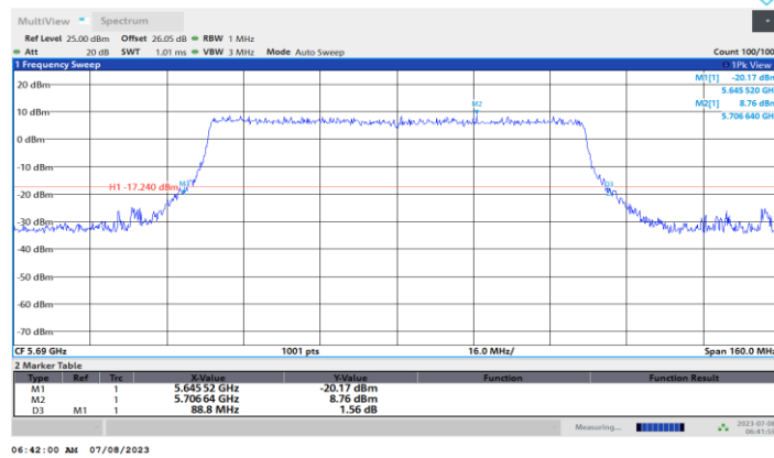
11BE80MIMO_Ant1_5690
