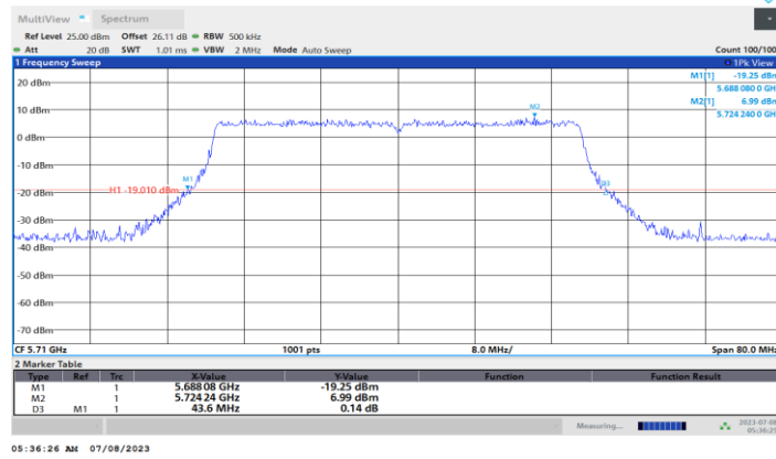
11BE40MIMO_Ant2_5710
