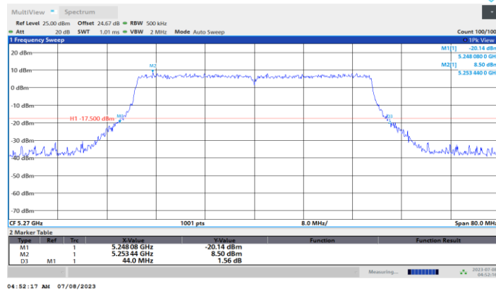
11BE40MIMO_Ant4_5270
