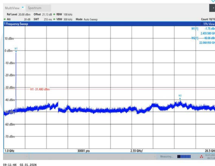
11N40MIMO_Ant2_2452_0~Reference
