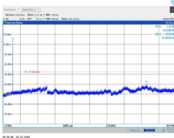
11N20MIMO_Ant2_2412_0~Reference
