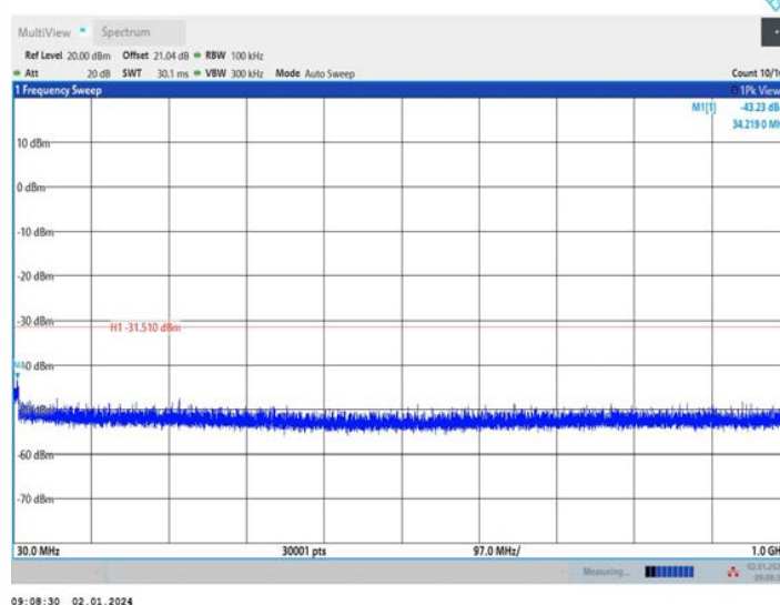
11N40MIMO_Ant2_2437_30~1000
