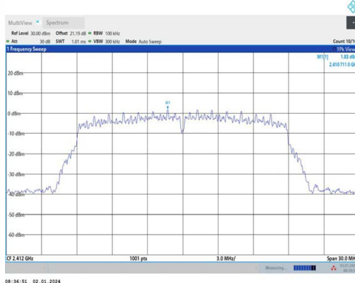
11N20MIMO_Ant2_2412_0~Reference
