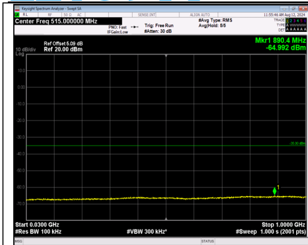
7-7-20MHz-20MHz-QPSK-QPSK-21001-21199-1RB#0-1 RB#99-30~1000MHz-PASS
