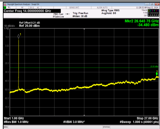
7-7-20MHz-10MHz-QPSK-QPSK-21251-21395-100RB#0-50RB#0-1000~27000MHz-PASS
