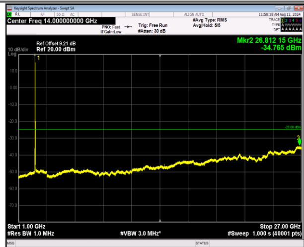
7-7-20MHz-20MHz-QPSK-QPSK-21152-21350-1RB#0-ORB #0-1000~27000MHz-PASS
