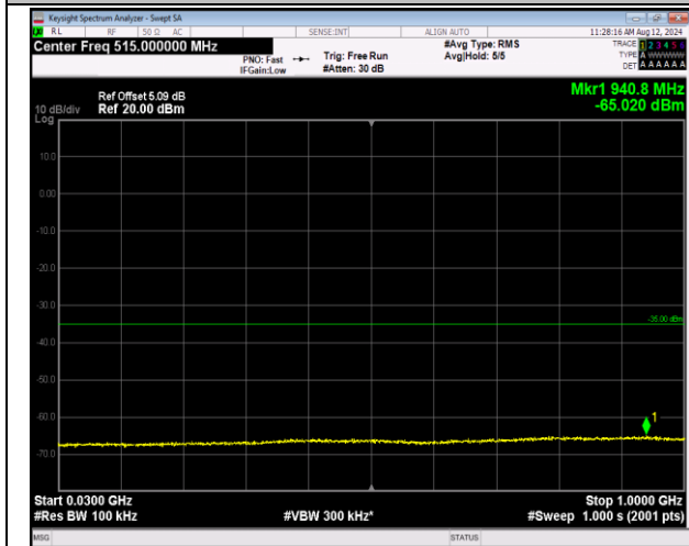
7-7-20MHz-10MHz-QPSK-QPSK-21251-21395-100RB#0-50RB#0-30~1000MHz-PASS
