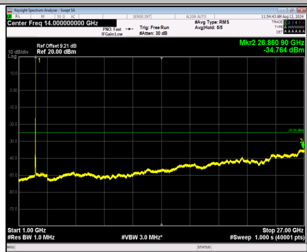
7-7-20MHz-20MHz-QPSK-QPSK-21001-21199-1RB#99-0R B#0-1000~27000MHz-PASS
