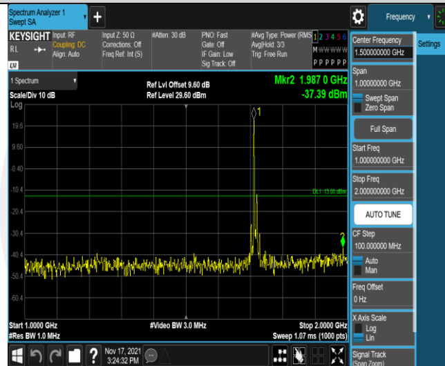
Band4-10MHz-QPSK-20000-1RB#0-Range2:1000~2000MHz
