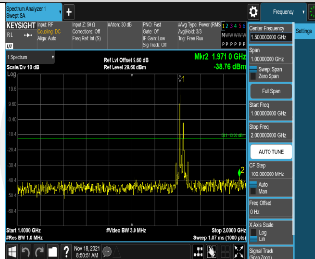
Band4-20MHz-QPSK-20050-1RB#0-Range2:1000~2000MHz
