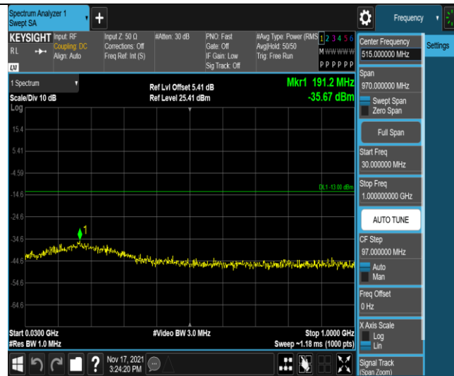
Band4-10MHz-QPSK-20000-1RB#0-Range1:30~1000MHz
