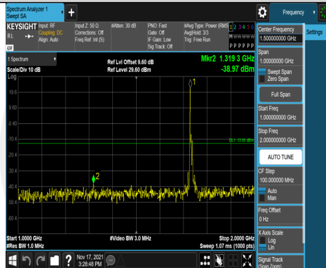
Band4-10MHz-QPSK-20175-1RB#0-Range2:1000~2000MHz
