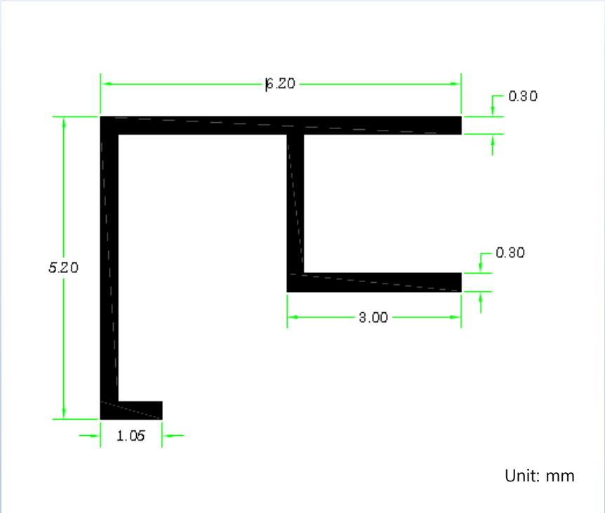
PCB Ant
