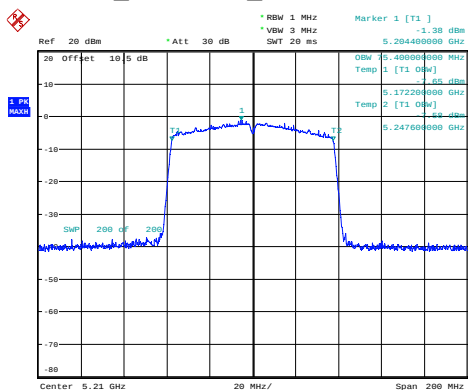
ac80_5210MHz_Chain 0 75.400MHz
