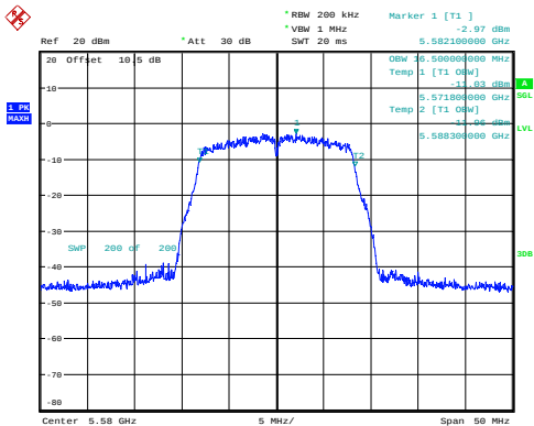
a_5580MHz_Chain 0 16.500MHz
