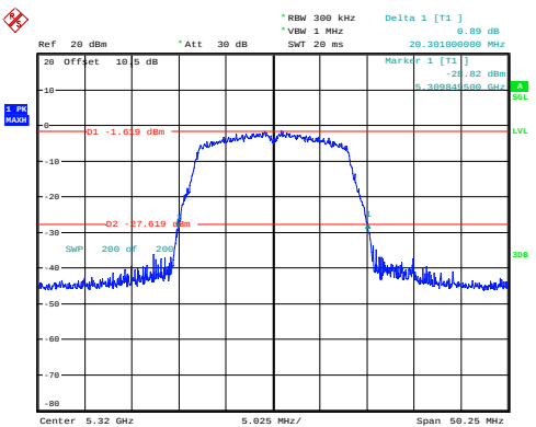
a_5320MHz_Chain 0 20.301MHz
