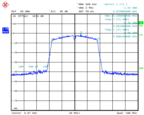
n40_5670MHz_Chain 0 36.200MHz
