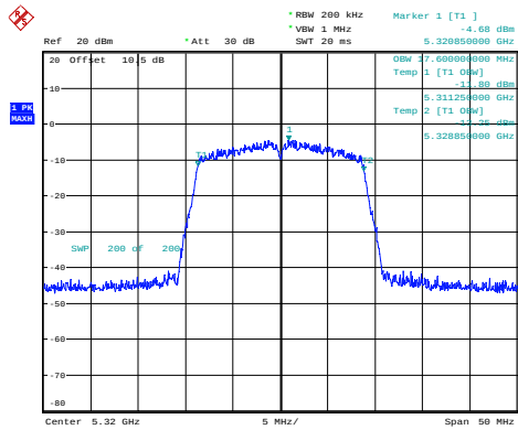
n20_5320MHz_Chain 0 17.600MHz
