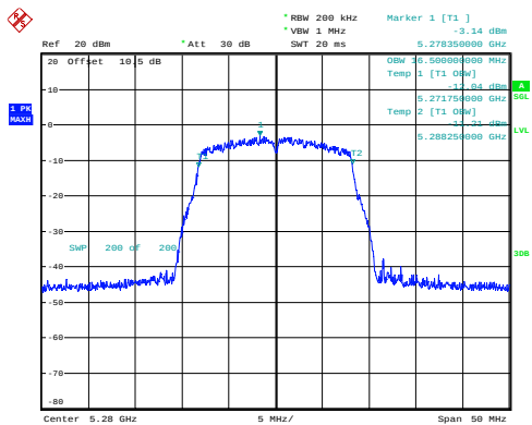
a_5280MHz_Chain 0 16.500MHz
