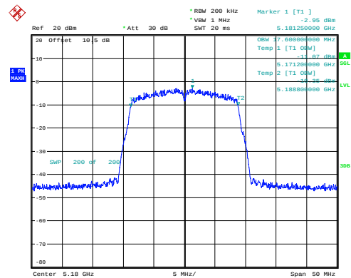
n20_5180MHz_Chain 0 17.600MHz
