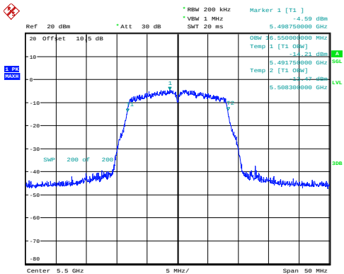
a_5500MHz_Chain 0 16.550MHz
