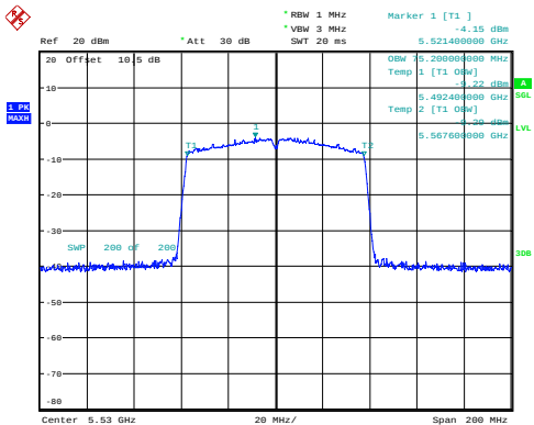
ac80_5530MHz_Chain 0 75.200MHz
