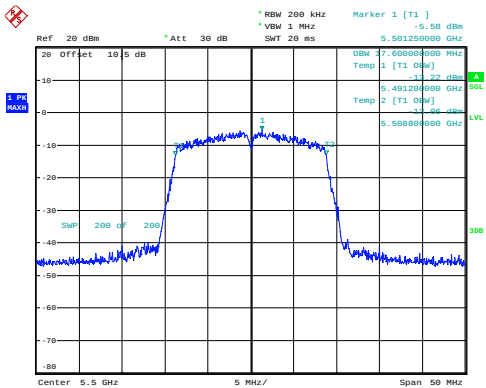
n20_5500MHz_Chain 0 17.600MHz
