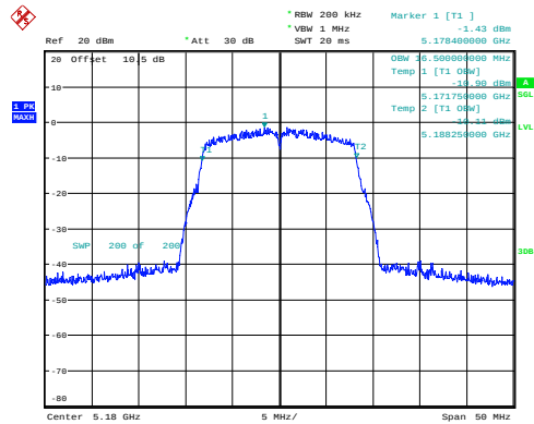
a_5180MHz_Chain 0 16.500MHz
