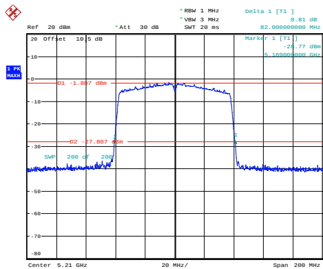
ac80_5210MHz_Chain 0 82MHz
