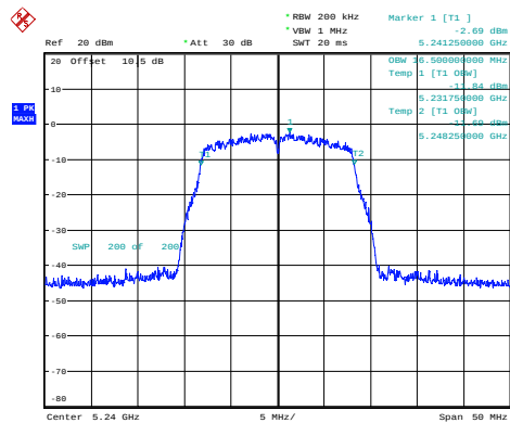
a_5240MHz_Chain 0 16.500MHz
