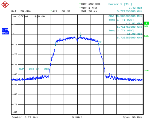
a_5720MHz_Chain 0 16.500MHz
