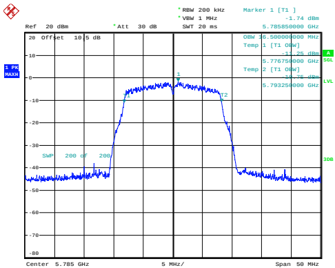
a_5785MHz_Chain 0 16.500MHz
