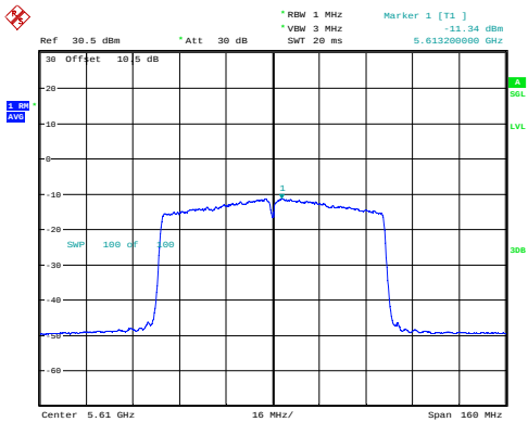
ac80_5610MHz_Chain 0 -11.34dBm/MHz
