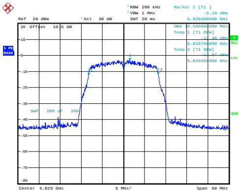
a_5825MHz_Chain 0 16.500MHz
