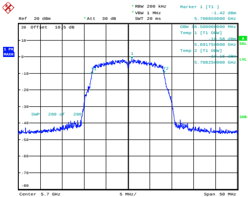
a_5700MHz_Chain 0 16.500MHz
