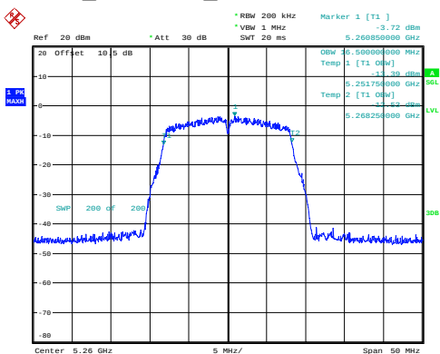
a_5260MHz_Chain 0 16.500MHz
