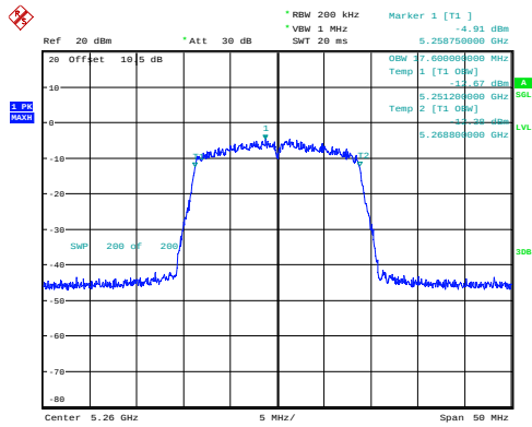
n20_5260MHz_Chain 0 17.600MHz
