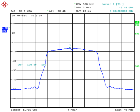
a_5785MHz_Chain 0 -6.48dBm/MHz
