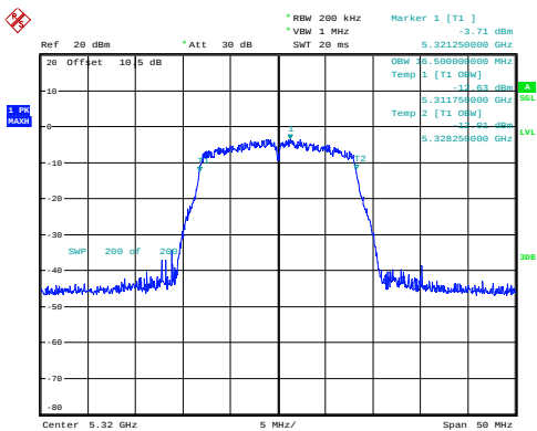
a_5320MHz_Chain 0 16.500MHz
