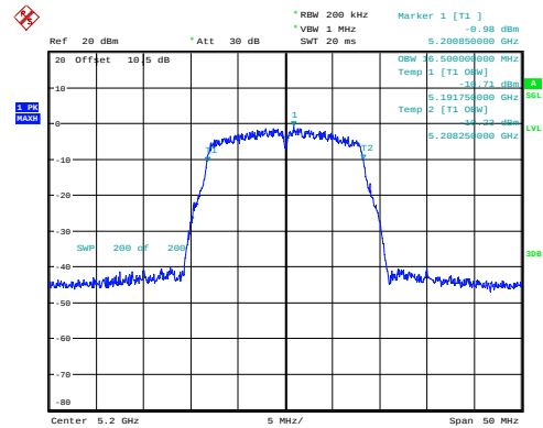
a_5200MHz_Chain 0 16.500MHz
