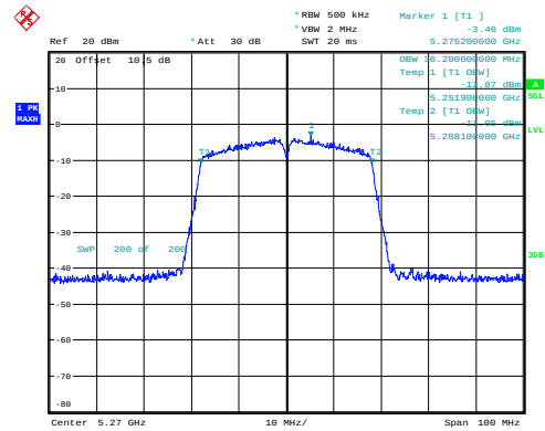
n40_5270MHz_Chain 0 36.200MHz
