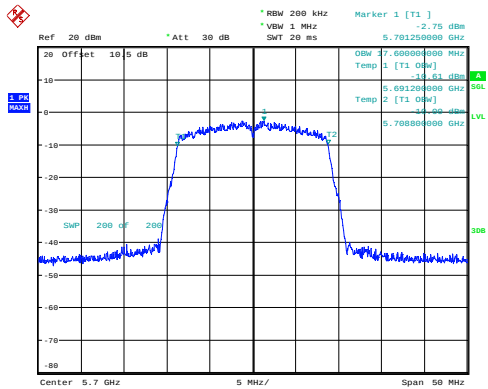
n20_5700MHz_Chain 0 17.600MHz
