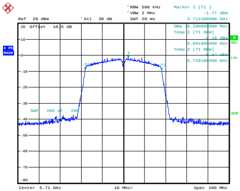
n40_5710MHz_Chain 0 36.200MHz
