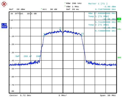
n20_5720MHz_Chain 0 17.600MHz
