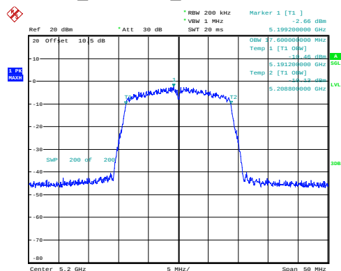
n20_5200MHz_Chain 0 17.600MHz
