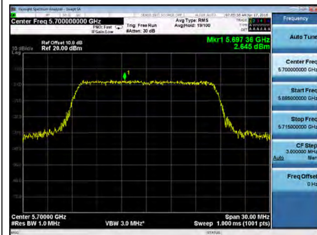
PSD-802.11a 5700MHz
