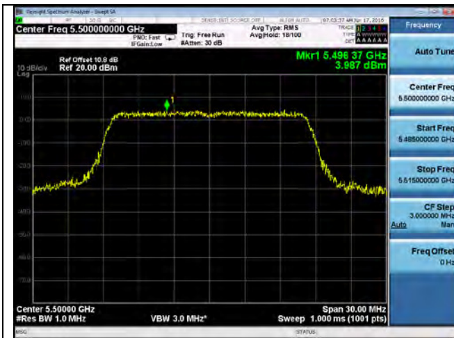
PSD-802.11a 5500MHz
