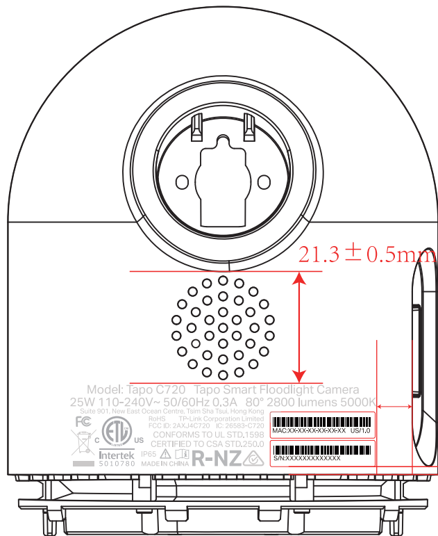
尺寸图
