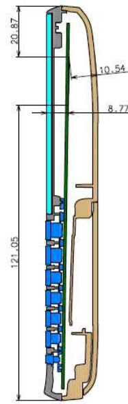
Sec. D-D (Pattern antenna)
