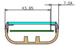
Sec. B-B (Pattern antenna)
