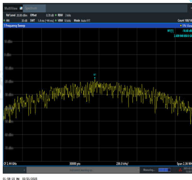
BLE 2M-Ant1-2440-PASS
