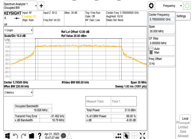
802.11ax_20MHz_Chain0_5785MHz
