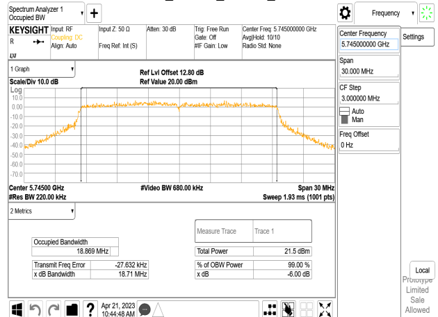
802.11ax_20MHz_Chain1_5745MHz
