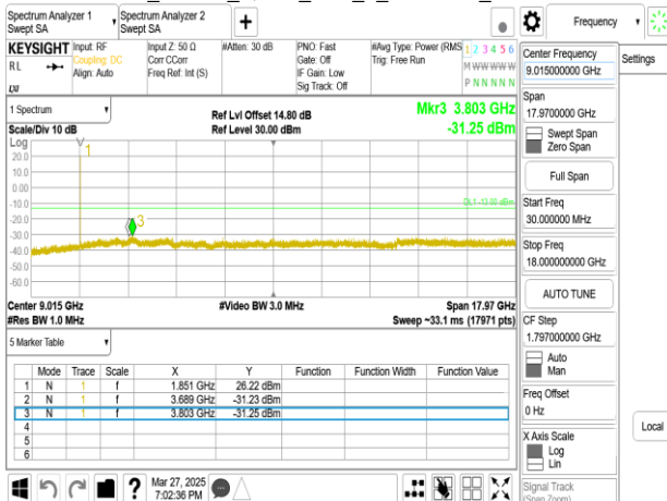
Band2_15MHz_QPSK_RB1_0_CH18675_upper 18G
