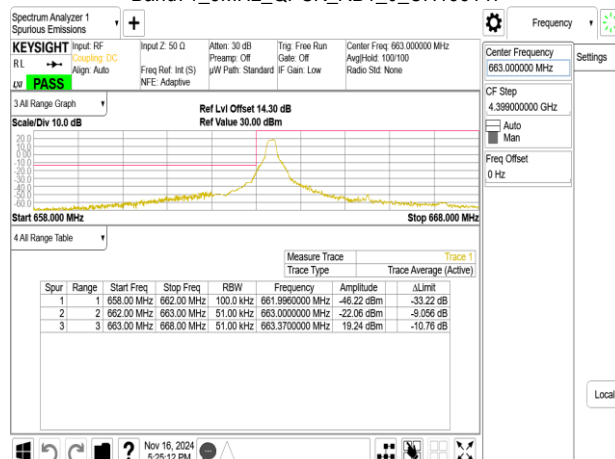
Band71_5MHz_QPSK_RB1_0_CH133147
