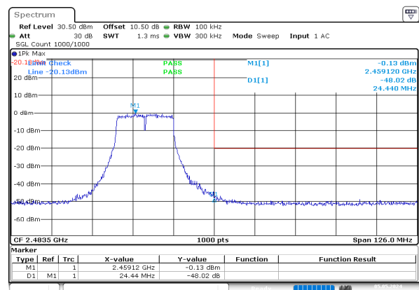
n20_2462MHz_Chain 0
