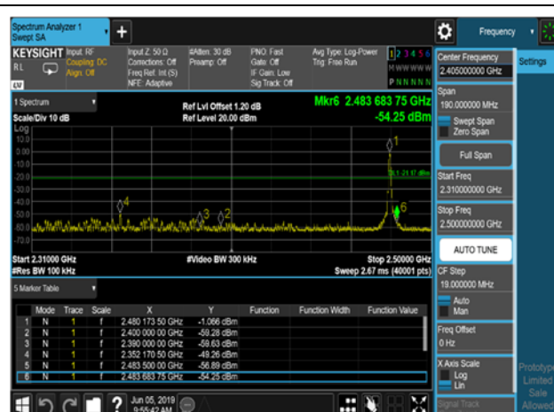
2480MHz,Plot 2,Band Edge
