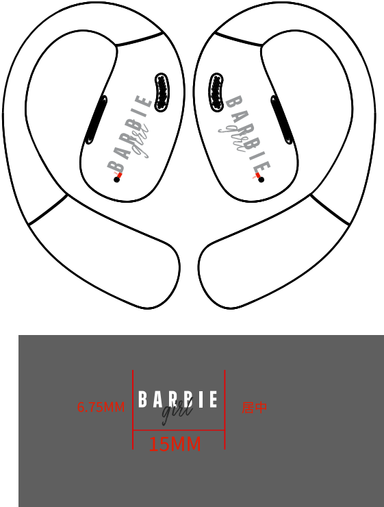
耳机正面
