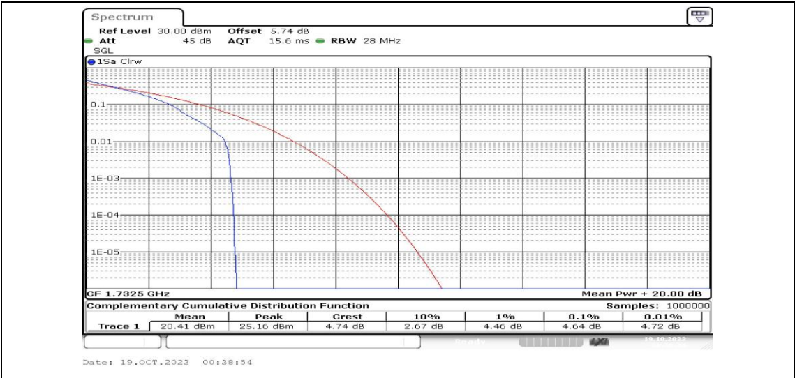
Band4-20MHz-QPSK-20175-1RB#0-PASS
