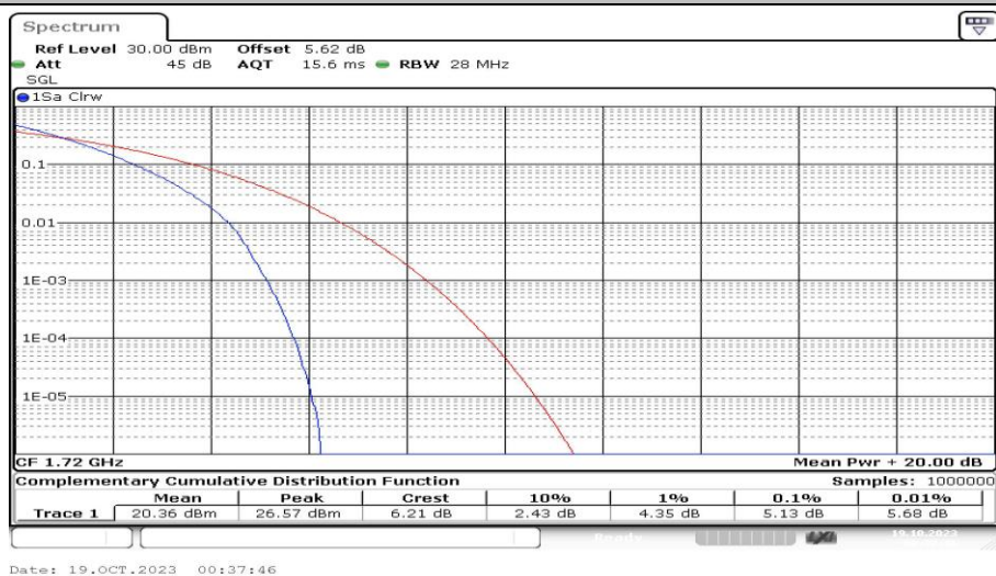
Band4-20MHz-QPSK-20050-100RB#0-PASS
