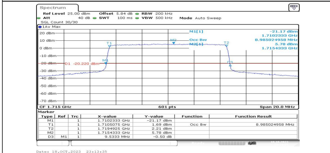
Band4-10MHz-QPSK-20000-50RB#0-PASS
