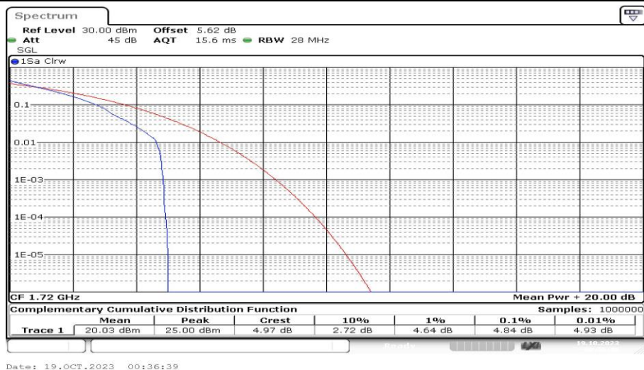
Band4-20MHz-QPSK-20050-1RB#0-PASS
