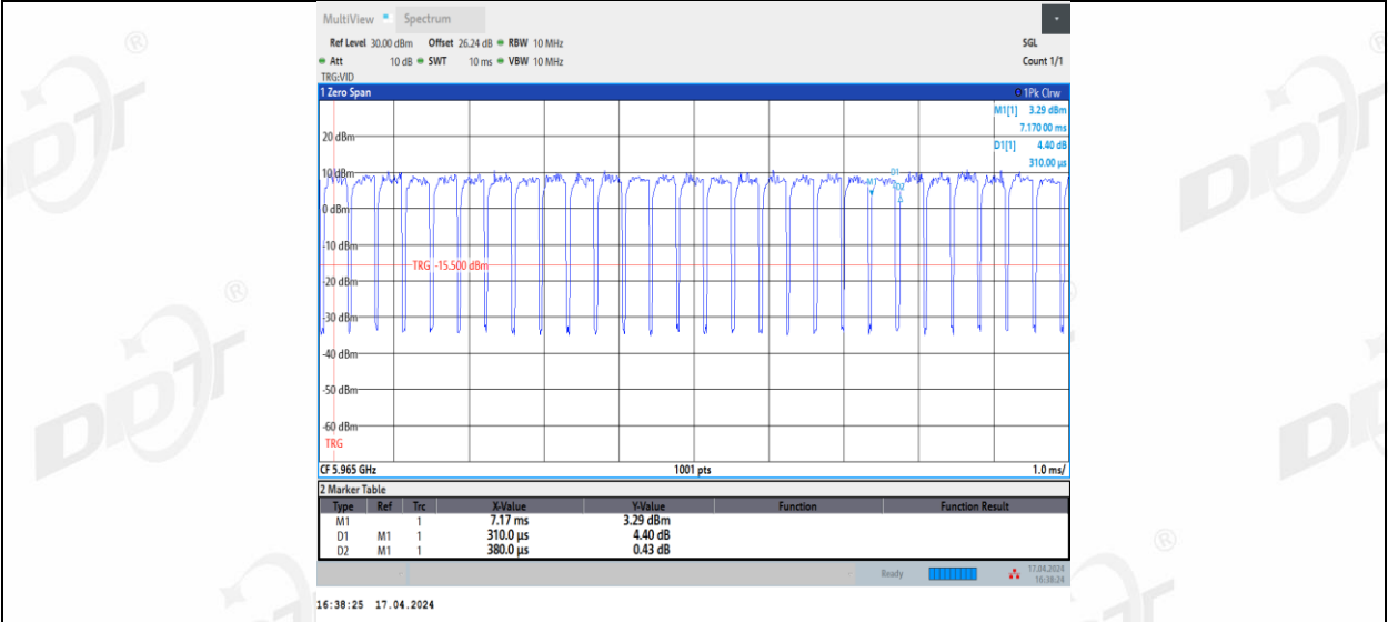
11AX40MIMO_Ant3_5965
