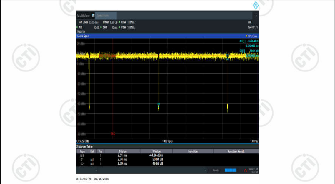
NTNV-11N20MIMO-Ant2-5220
