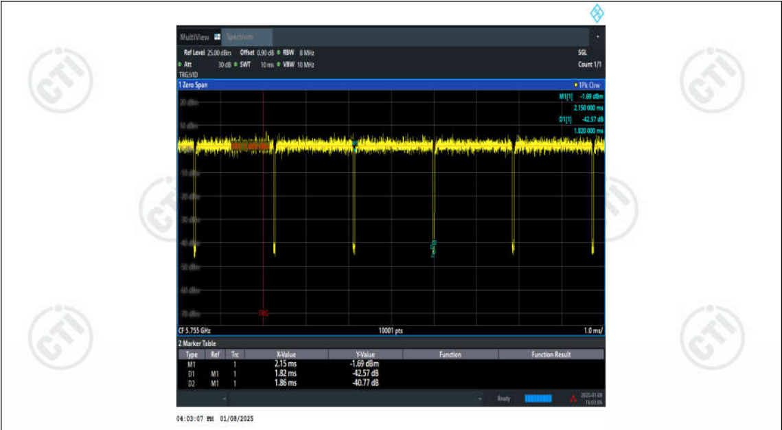
NTNV-11N40MIMO-Ant1-5755
