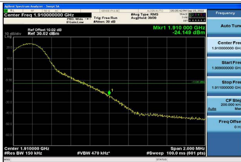
Band2-15MHz-16QAM-19125-1RB#74
